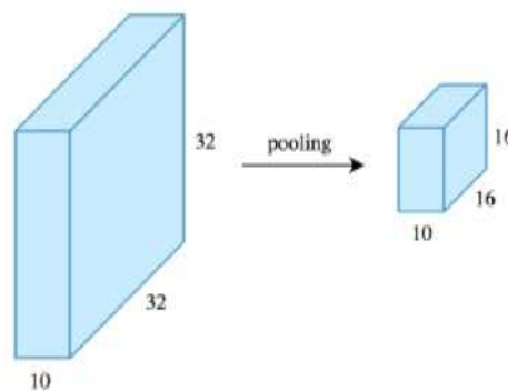
Fig. 3 Pooling layer
