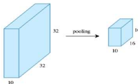
Fig. 3 Pooling layer
